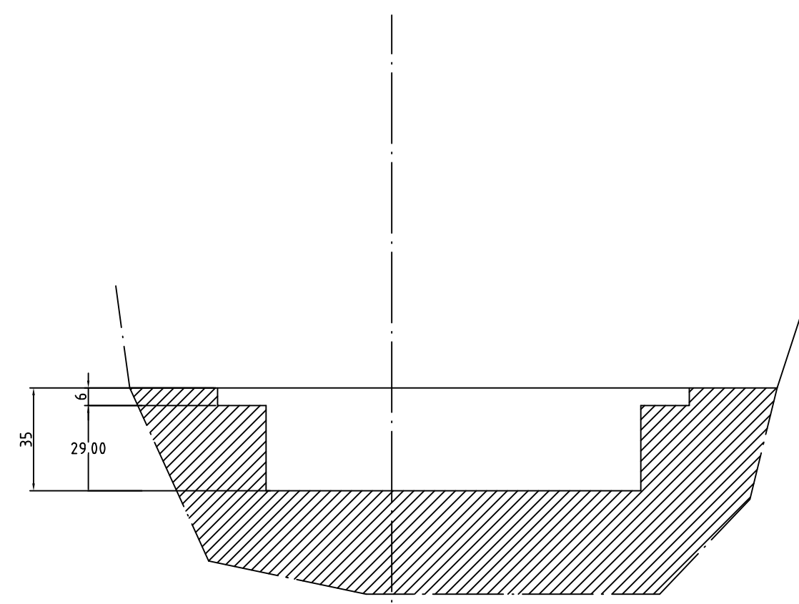
INCASSO CERNIERA SUPERIORE
